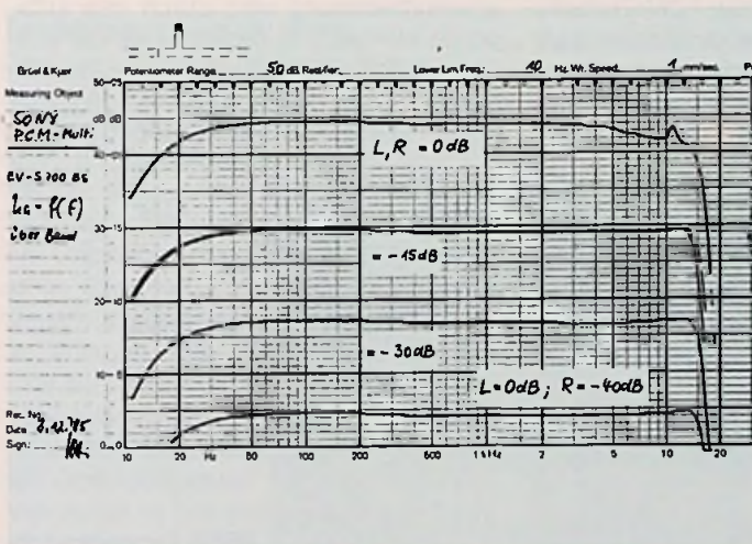
Bild 3: Übertragungsbereich und Frequenzgang einer PCM-Tonaufzeichnung auf V8-Videorecorder (Sony EV-S700ES)
