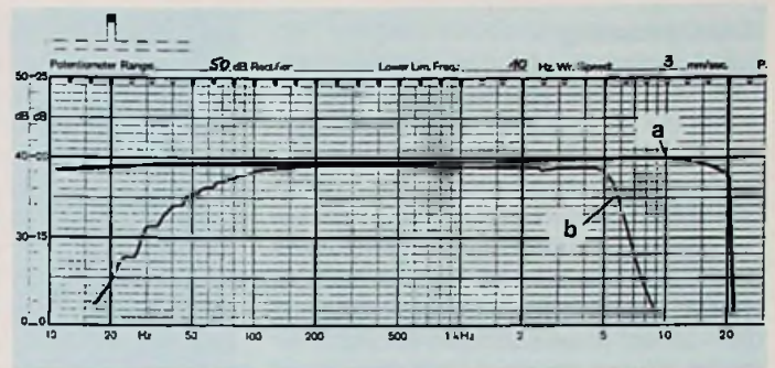
Bild 2: Deckungsgleiche Frequenzgänge bei einer HiFi-Schrägspuraufzeichnung mit normaler und halbiert Bandgeschwindigkeit (a) und reduzierter Übertragungsbereich des gleichzeitig aufgezeichneten Summensignals L + R in der klassischen Längsspur bei Longplay (b)
