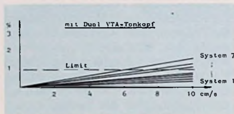
Bild 7: Einfluß der Schnelle auf die Verzerrungen beim VTA-Tonkopf mit Spurwinkelkorrektur
