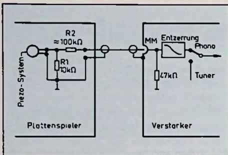
Bild 1: Piezo-Tonabnehmer am Eingang für magnetische Tonabnehmer
