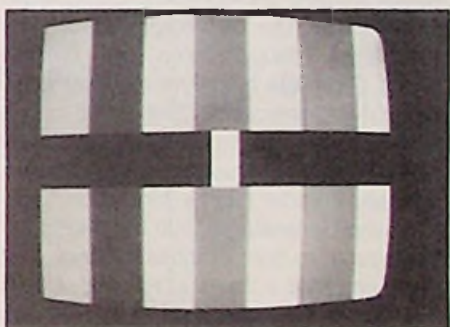
Bild 7: Das „bewegte Testbild“ eingeblendet in die Farbbalken
