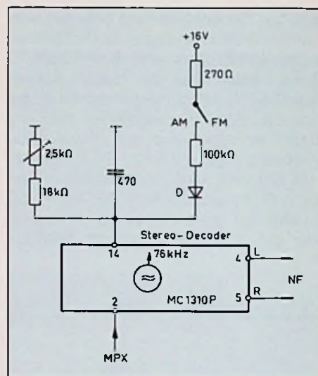
Bild 1: Die defekte Diode schaltete den Stereodecoder nicht ab
